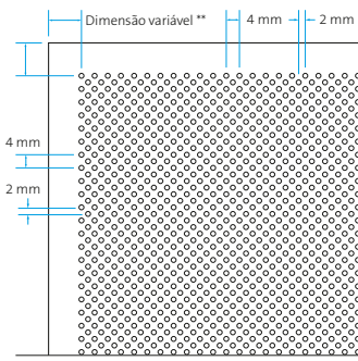
Perfuração Ø 1,5 mm Área perfurada ~ 22%
