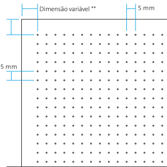
Perfuração ultra-micro Ø 0,7 mm Área perfurada ~ 1,5%
