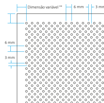
Perfuração Ø 2 mm Área perfurada ~ 18%
