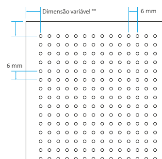
Perfuração Ø 2 mm Área perfurada ~ 9%
