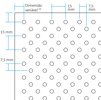
Perfuração Ø 4 mm Área perfurada ~ 11%
