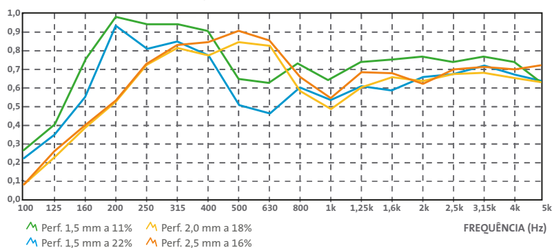
COEFICIENTE DE ABSORÇÃO \alpha_s
