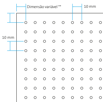
Perfuração Ø 2,5 mm Área perfurada ~ 5%
